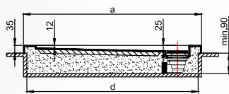
Flat h:3,5 cm Section A-A
